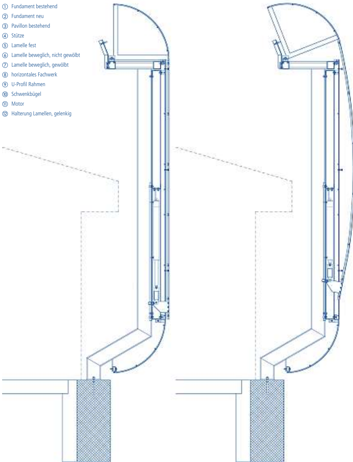
4 Vertikalschnitte Lamellen
